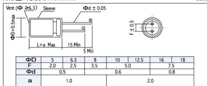
外形图尺寸表 Dimensions
